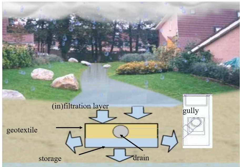
Schematische weergave van een wadi.
